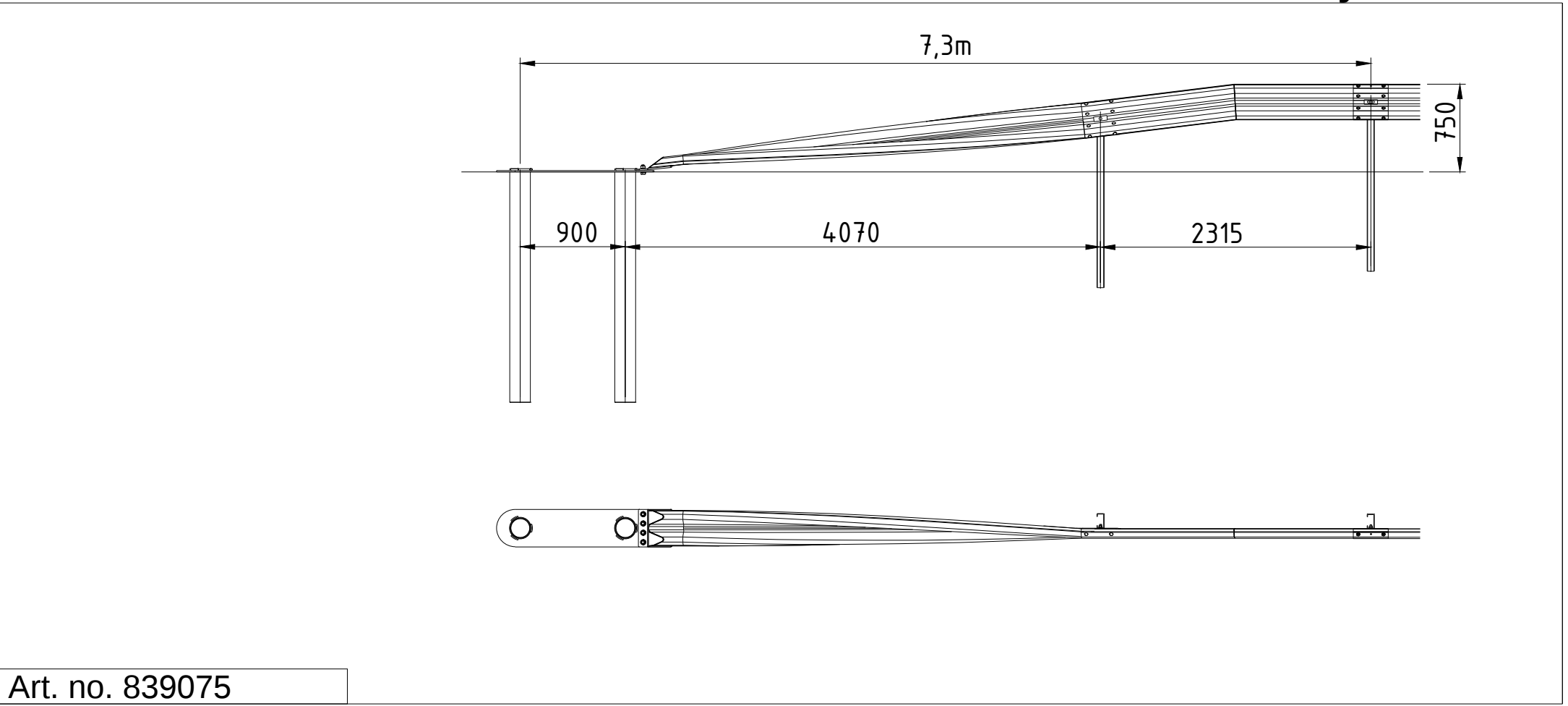
Förankring - Megarail EO - Avfart 7,3m - justerbar
