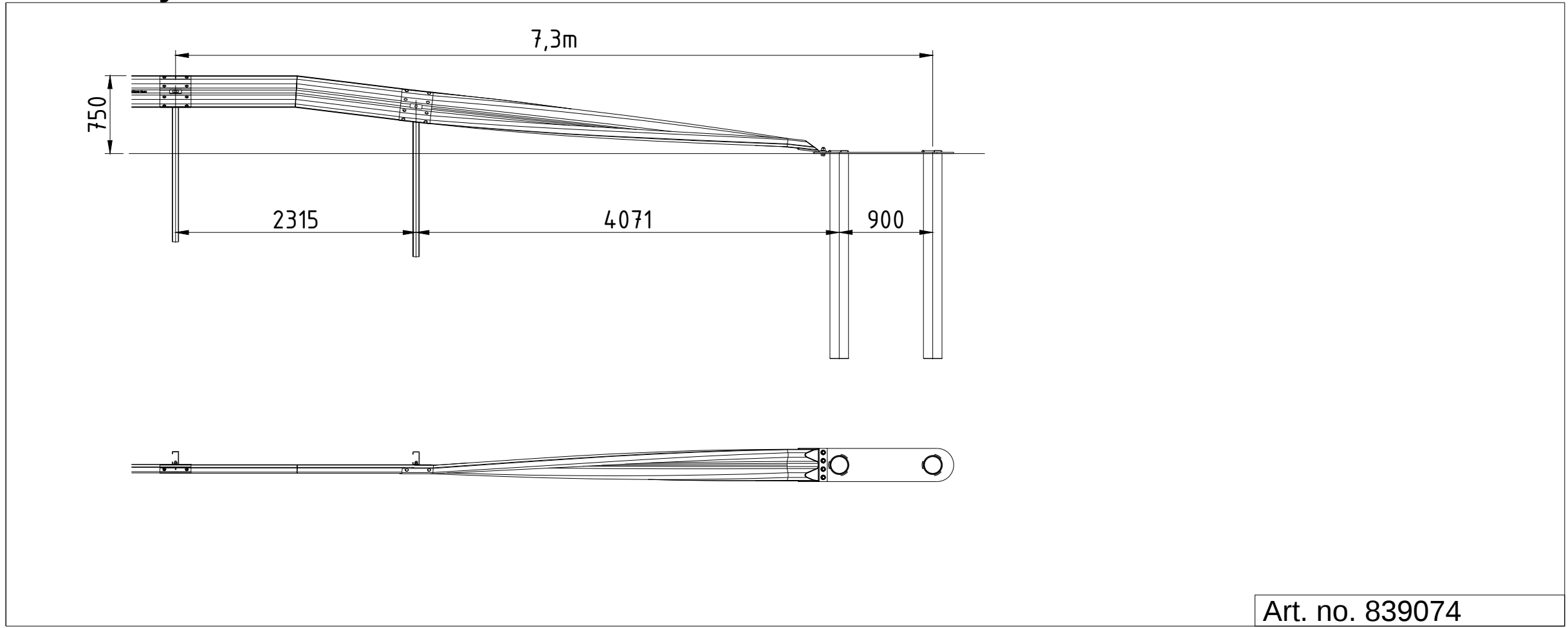
Förankring - Megarail EO - Påfart 7,3m - justerbar
