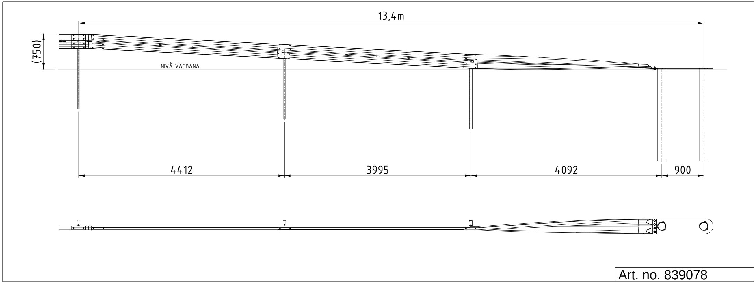
Förankring - Megarail EO - Påfart 13,4m - justerbar
