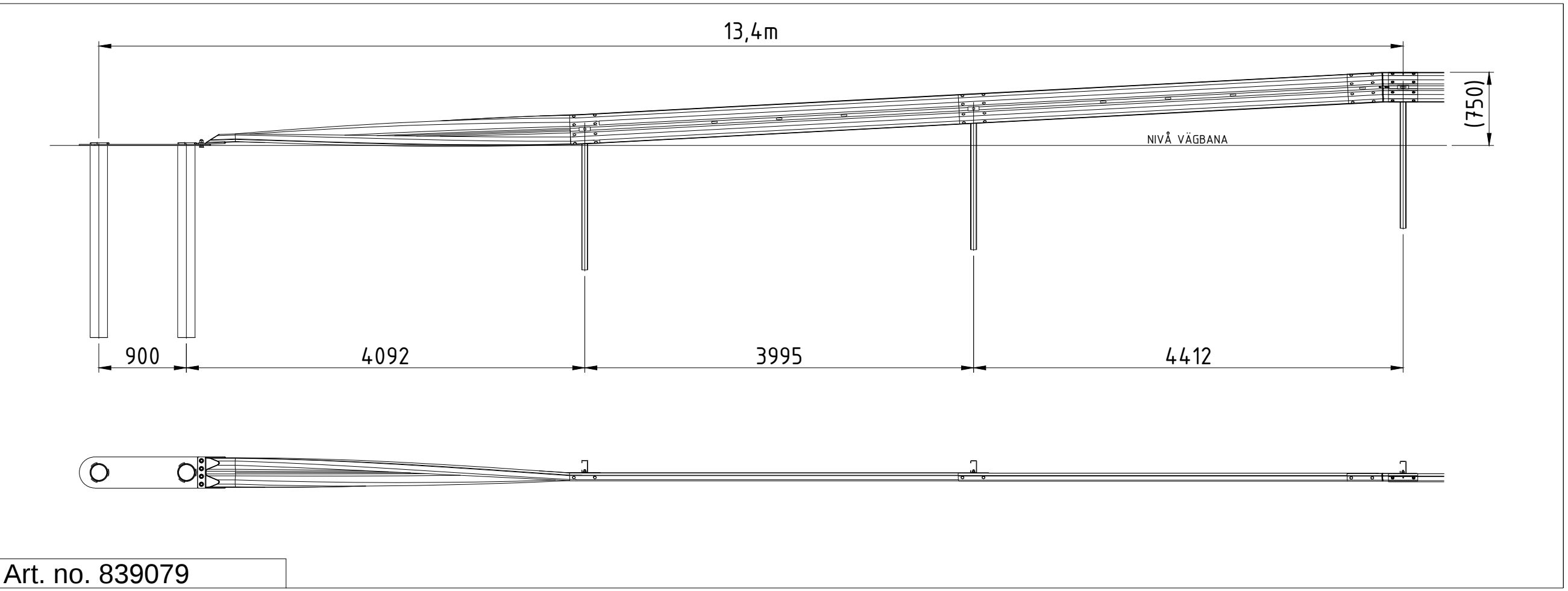
Förankring - Megarail EO - Avfart 13,4 - justerbar
