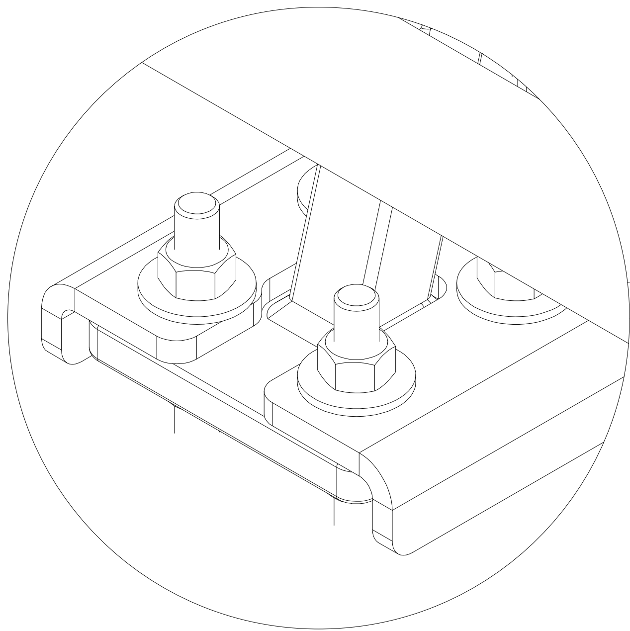
B ( 1 : 2 ) INFÄSTNING BULTGRUPP
