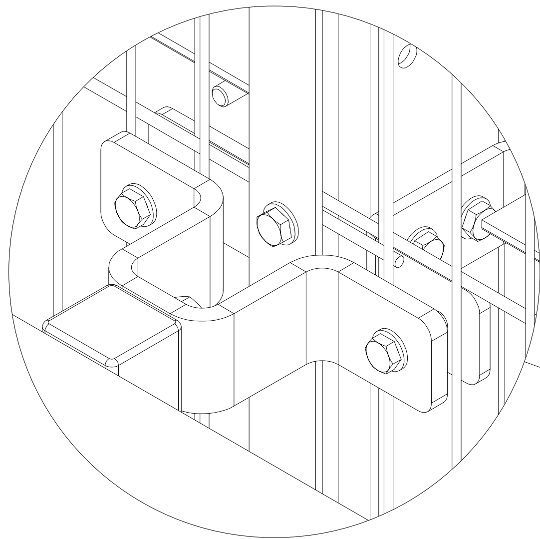
A ( 1 : 2 ) INFÄSTNING RÄCKESTÅNDARE
