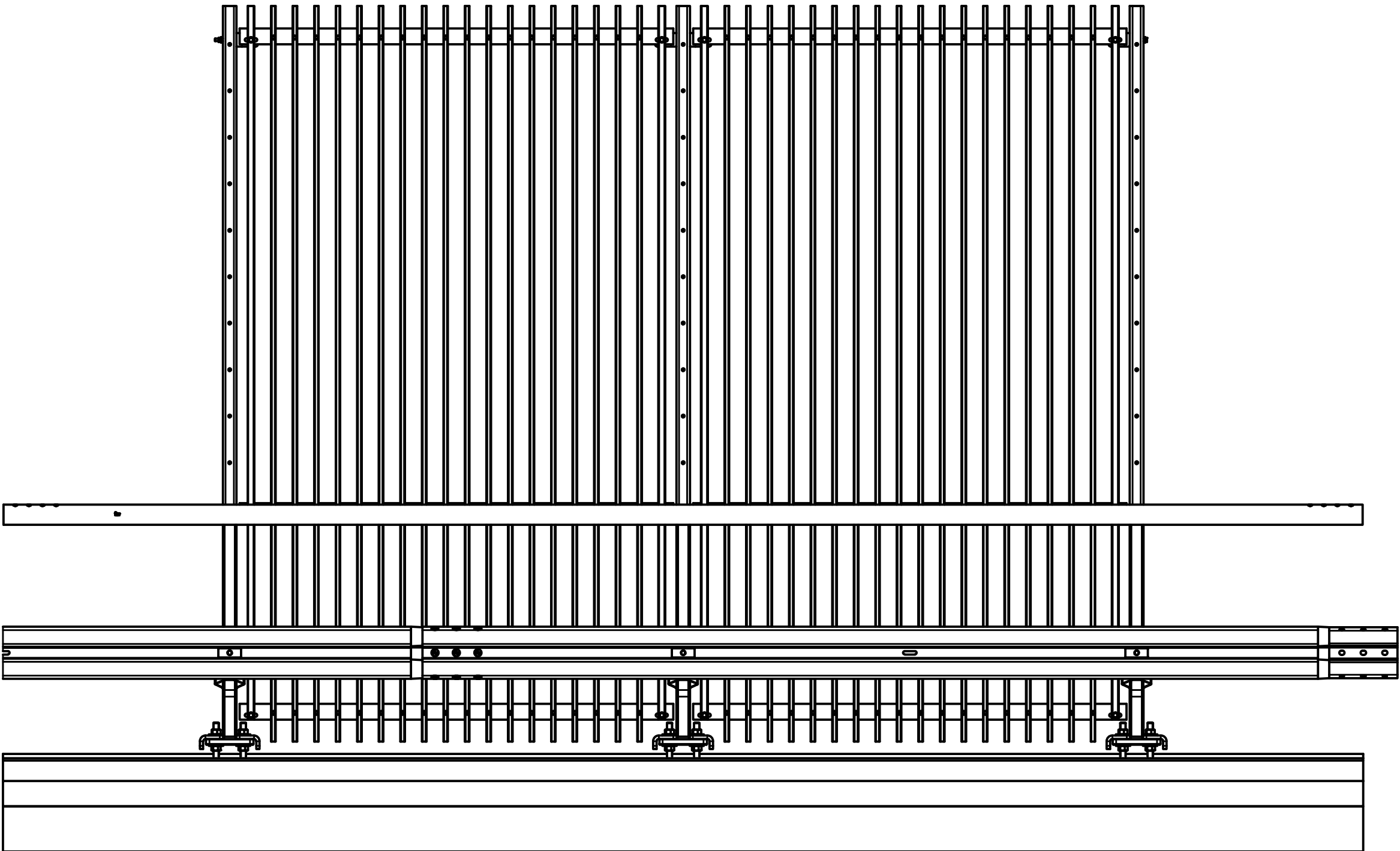
BIRSTA SP MED SUICIDSKYDD (SPJÄLOR) ARTIKELNUMMER 839206-n / 839206-nL ( 1 : 20 )
