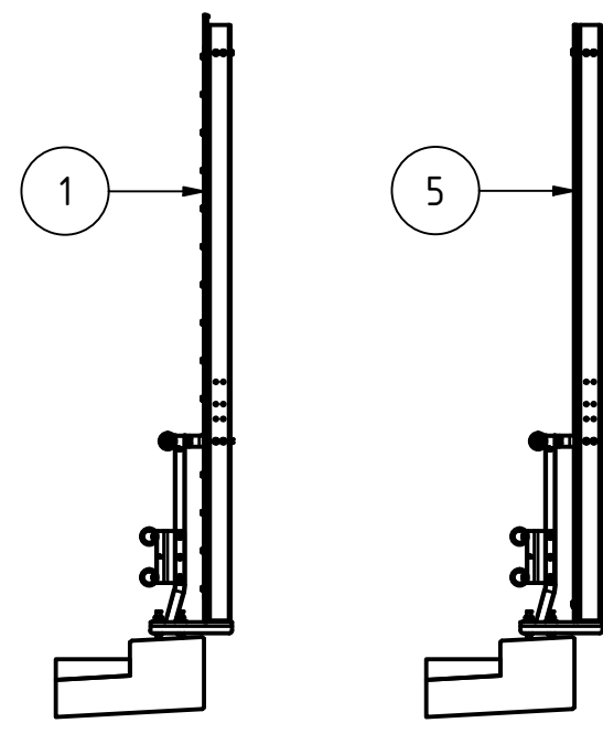
KANTBALK A, RÄCKESHÖJD 1220 MM
