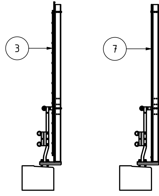
KANTBALK B, RÄCKESHÖJD 1220 MM
