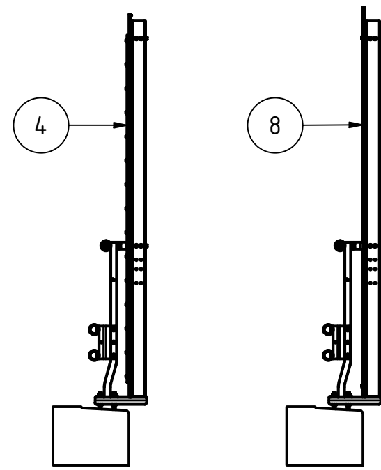
KANTBALK B, RÄCKESHÖJD 1420 MM
