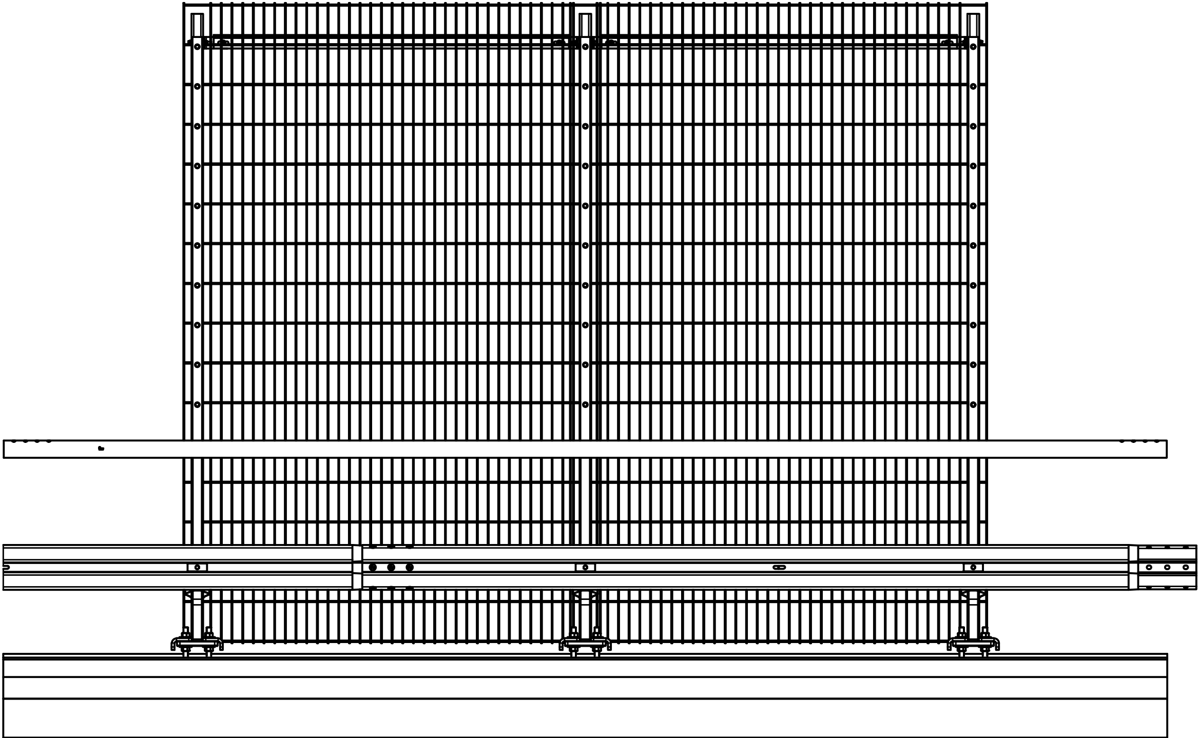
BIRSTA SP MED SUICIDSKYDD (NÄT) ARTIKELNUMMER 839205-n / 839205-nL ( 1 : 20 )
