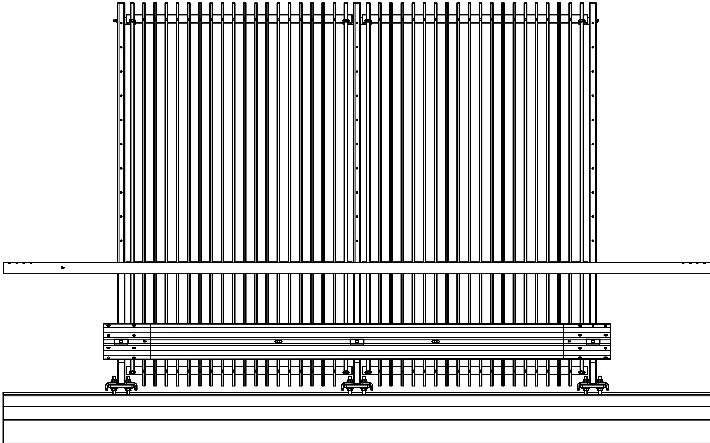
BIRSTA WP MED SUICIDSKYDD (SPJÄLOR) ARTIKELNUMMER 839203-n / 839203-nL ( 1 : 20 )
