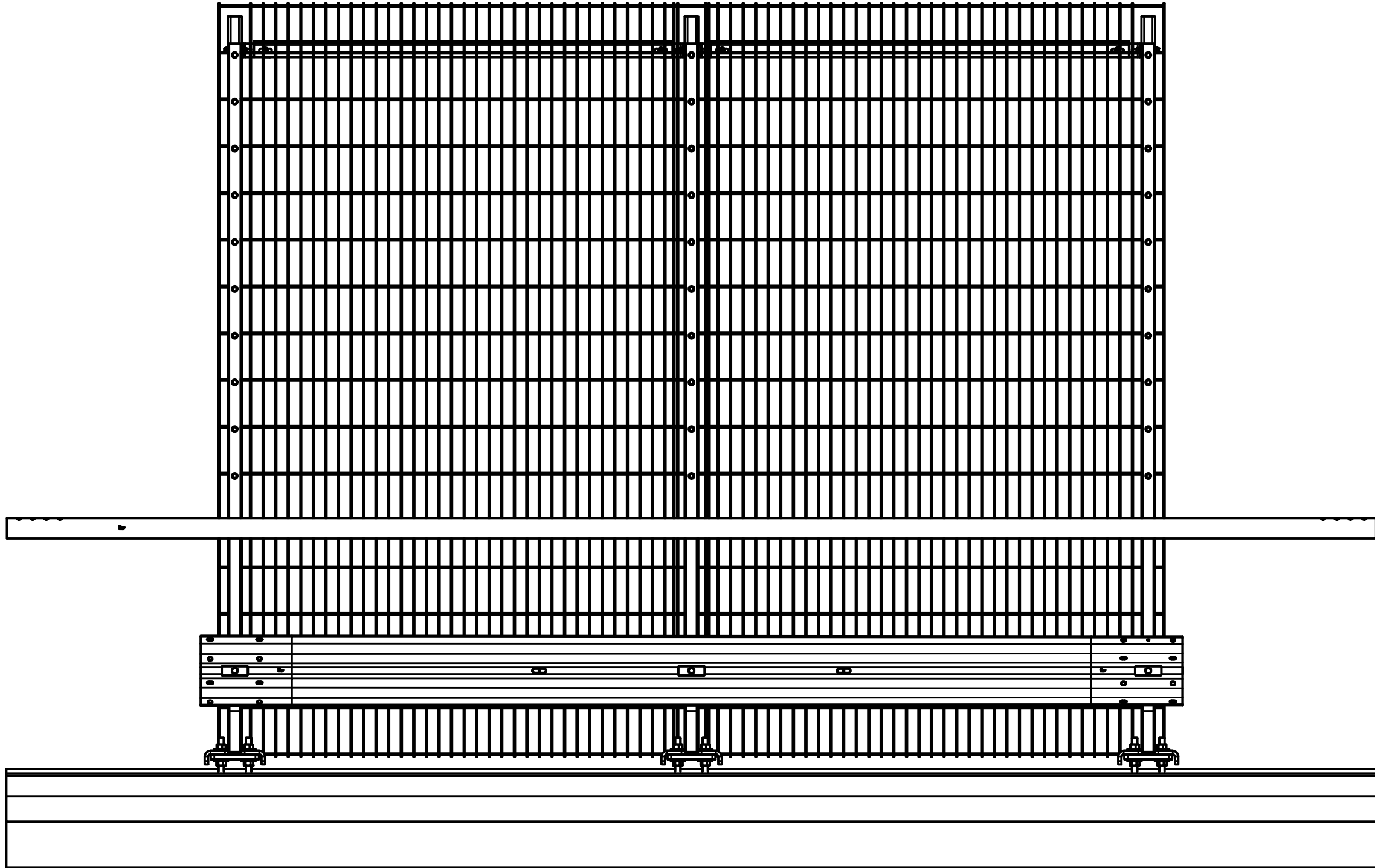
BIRSTA WP MED SUICIDSKYDD (NÄT) ARTIKELNUMMER 839202-n / 839202-nL ( 1 : 20 )
