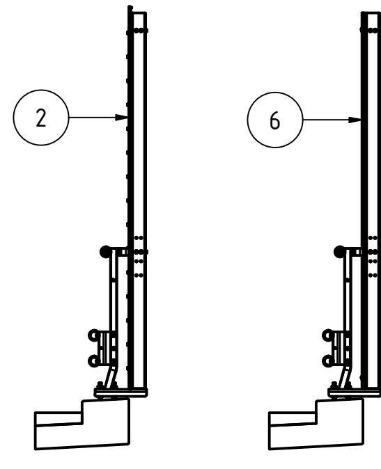
KANTBALK A, RÄCKESHÖJD 1420 MM
