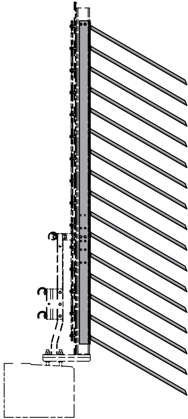
KANTBALK B, RÄCKESHÖJD 1220 MM ( 1 : 20 )
