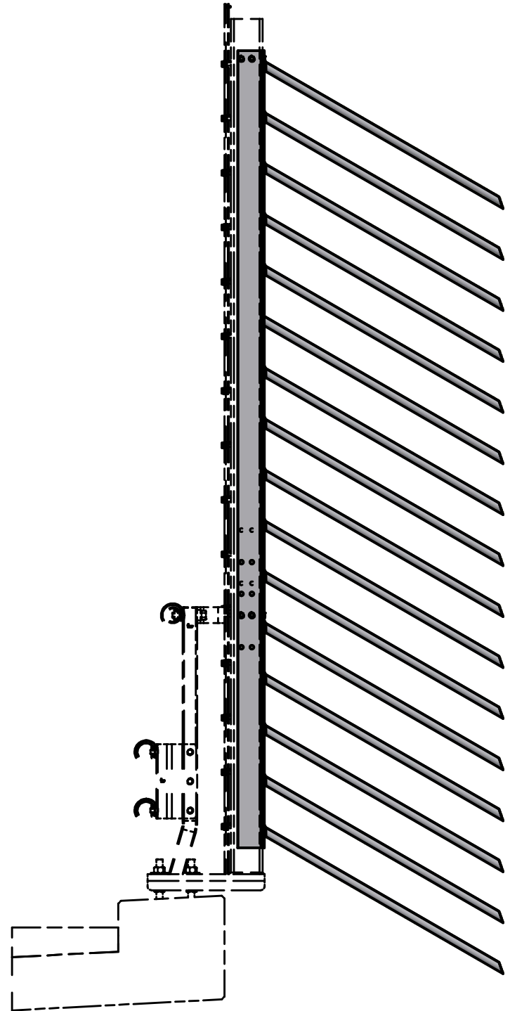
KANTBALK A, RÄCKESHÖJD 1220 MM ( 1 : 20 )
