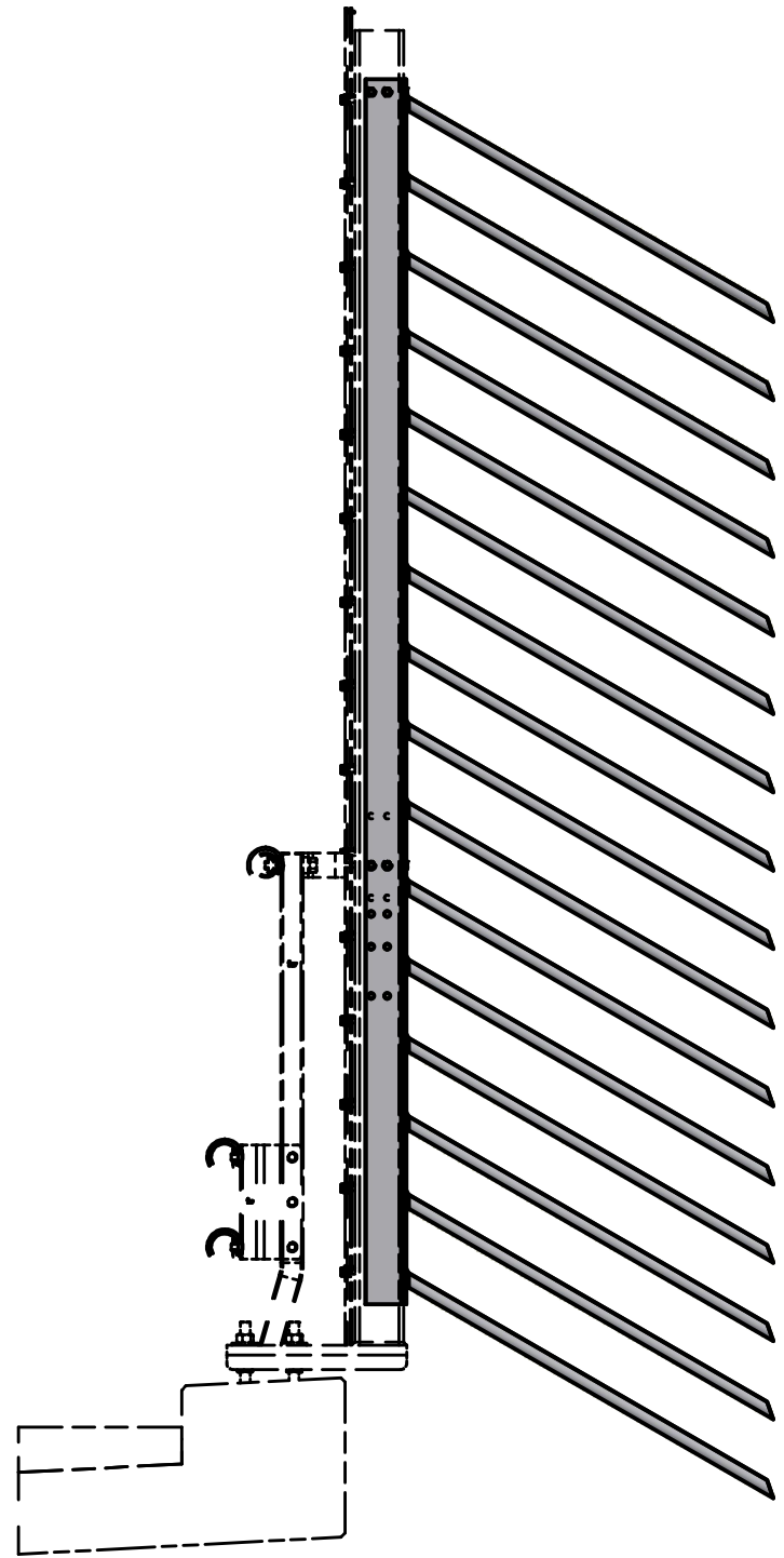
KANTBALK A, RÄCKESHÖJD 1420 MM ( 1 : 20 )
