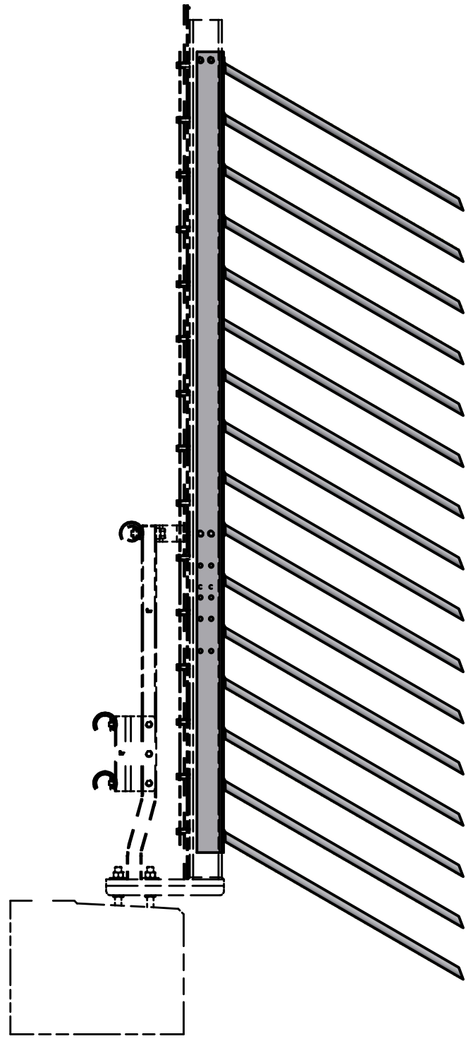
KANTBALK B, RÄCKESHÖJD 1420 MM ( 1 : 20 )
