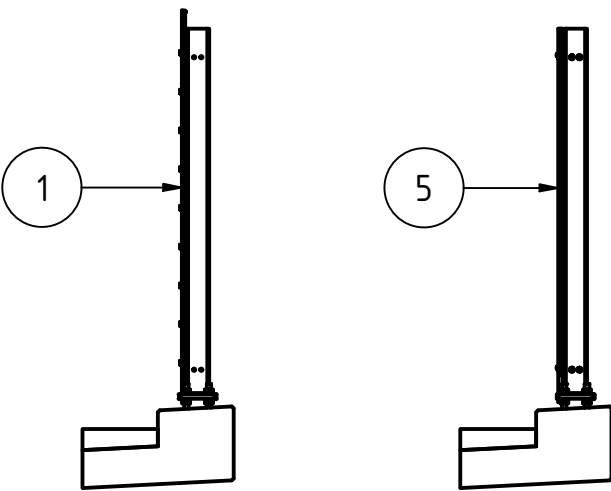
KANTBALK A, OVANPÅ
