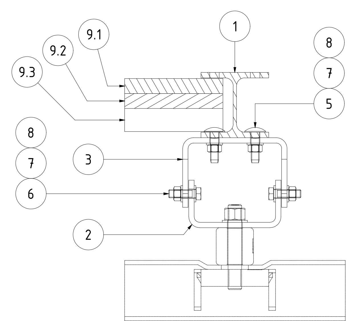
A-A ( 1 : 3 )
