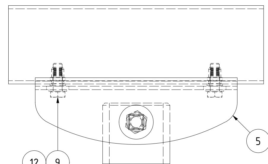
D ( 1 : 2 )
