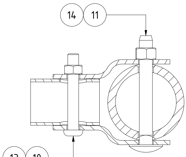
H-H ( 1 : 2 )
