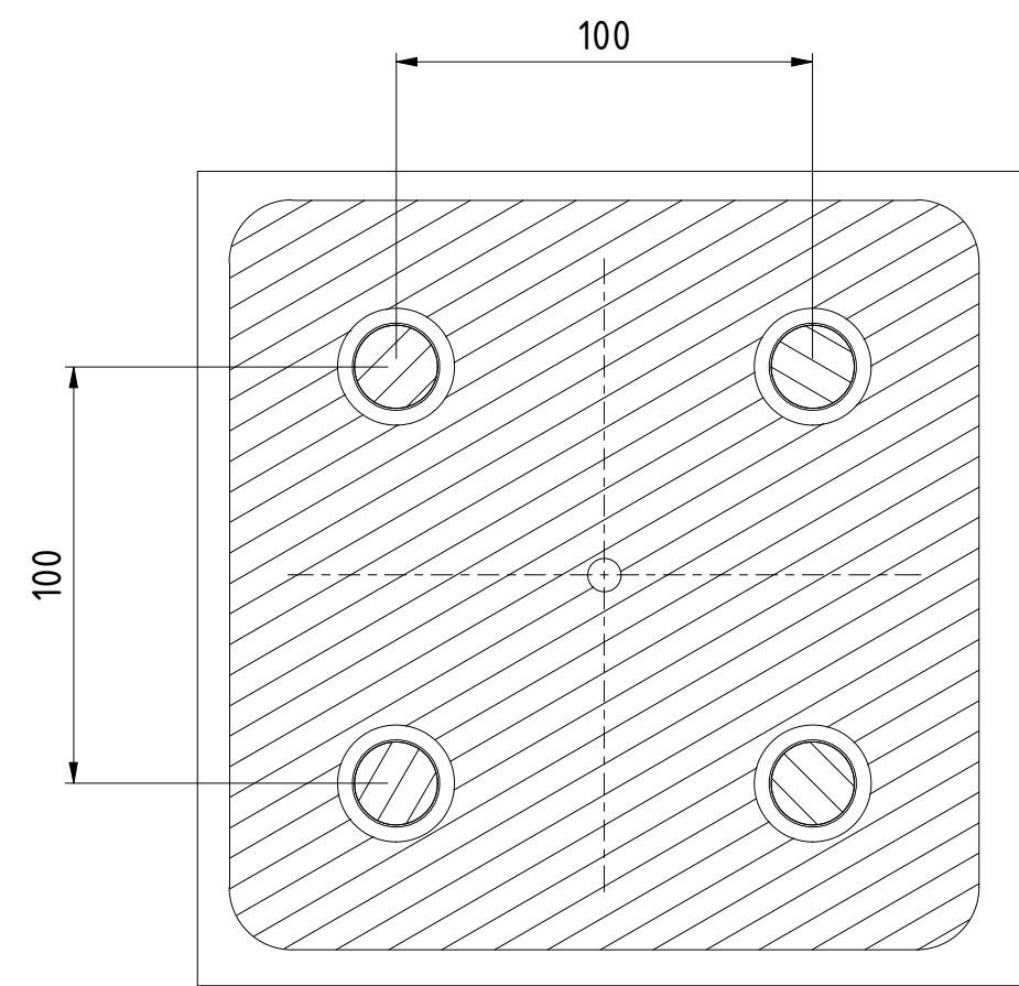
G-G ( 1 : 2 )
