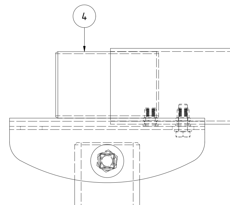
E ( 1 : 2 )
