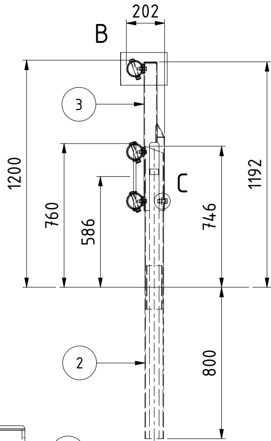
A-A ( 1 : 20 )
