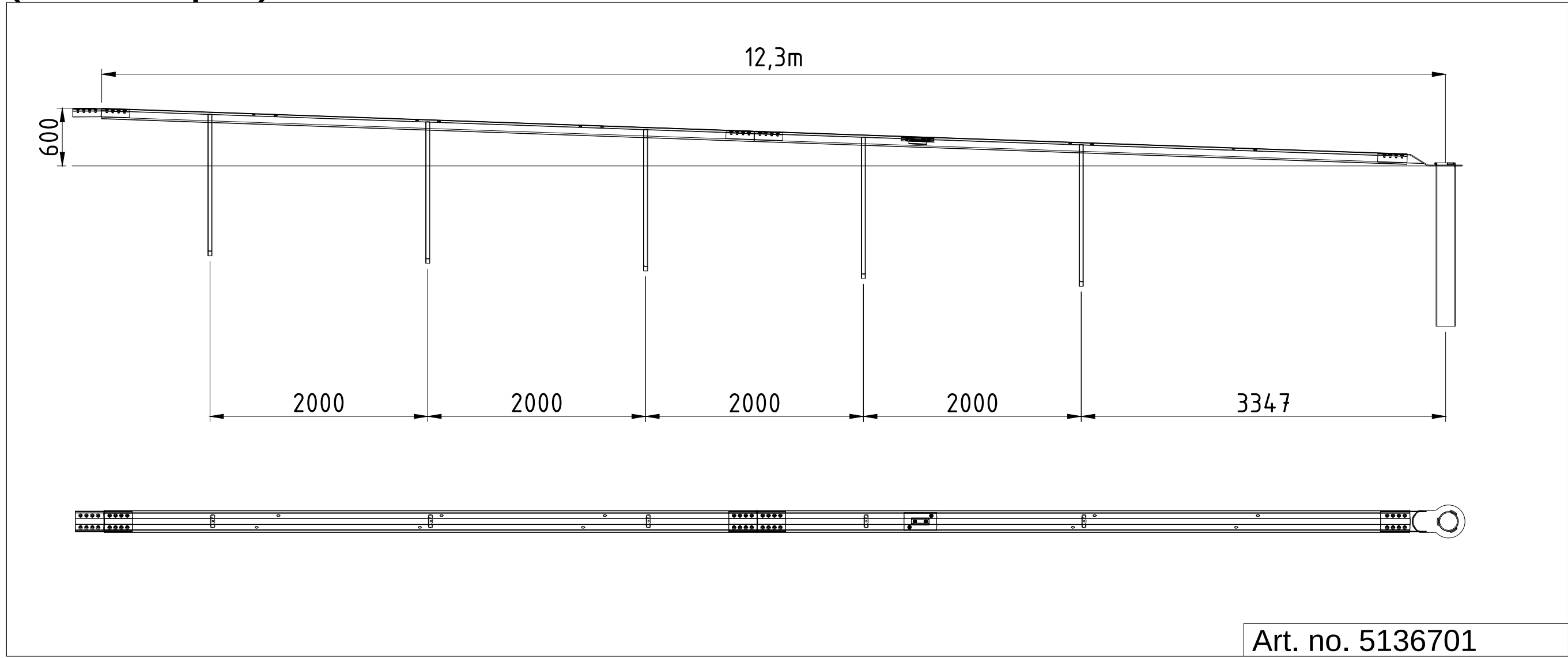
Förankring - Safeline-M - Påfart / Avfart 12,3m (1,5m Spik)
